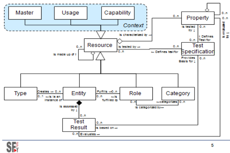
Fig. . Resource meta-model
